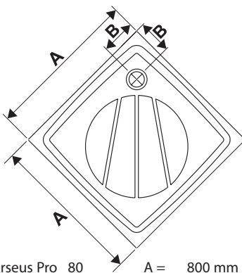
Perseus Pro 80 A = 800 mm Perseus Pro 90 A = 900 mm Perseus Pro 100 A = 1000 mm B = 200 mm
